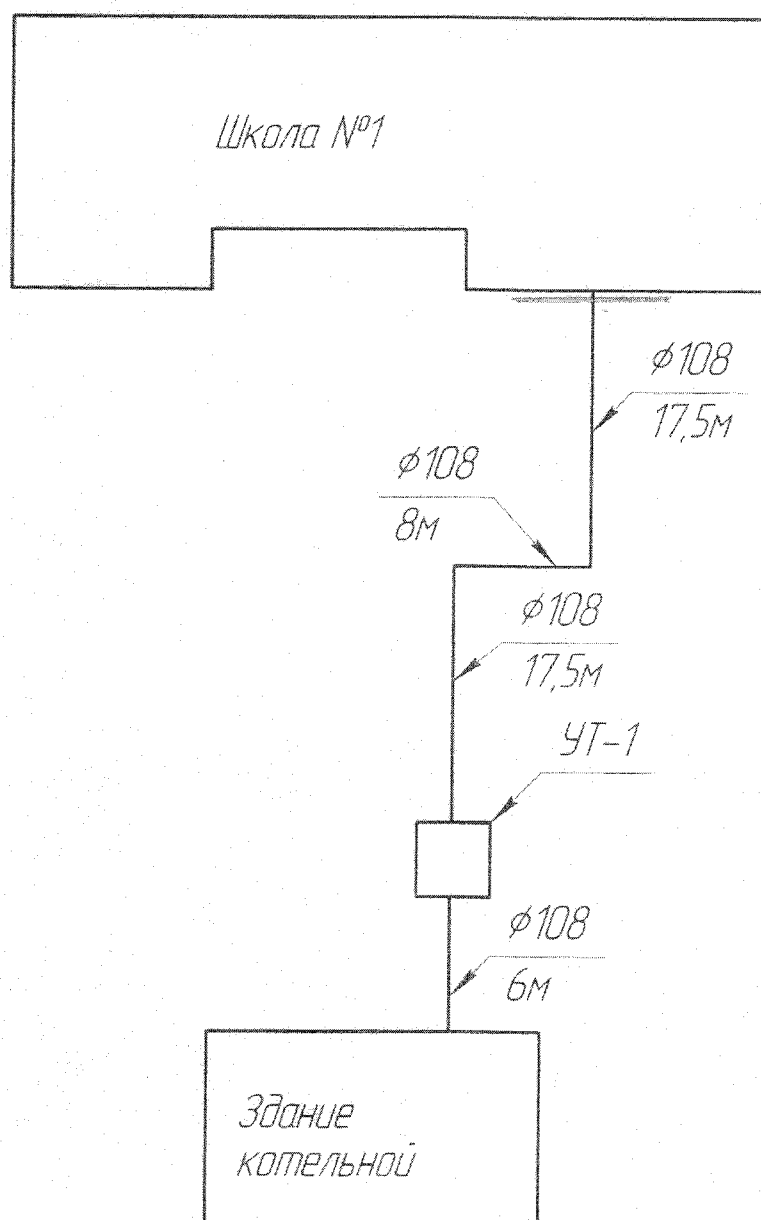
Схема тепловой сети МКОУ "СОШ №1" п. Пристен ул. Почтовая
